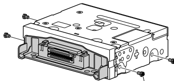
Vis à tête hexagonale x 4
